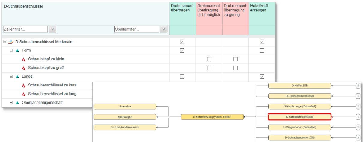
Abb.: Verknüpfungsmatrix für Systeme, Funktionen und Fehler sowie Visualisierung als Netzdarstellung
